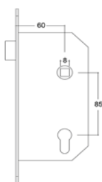
Fechadura trinco
